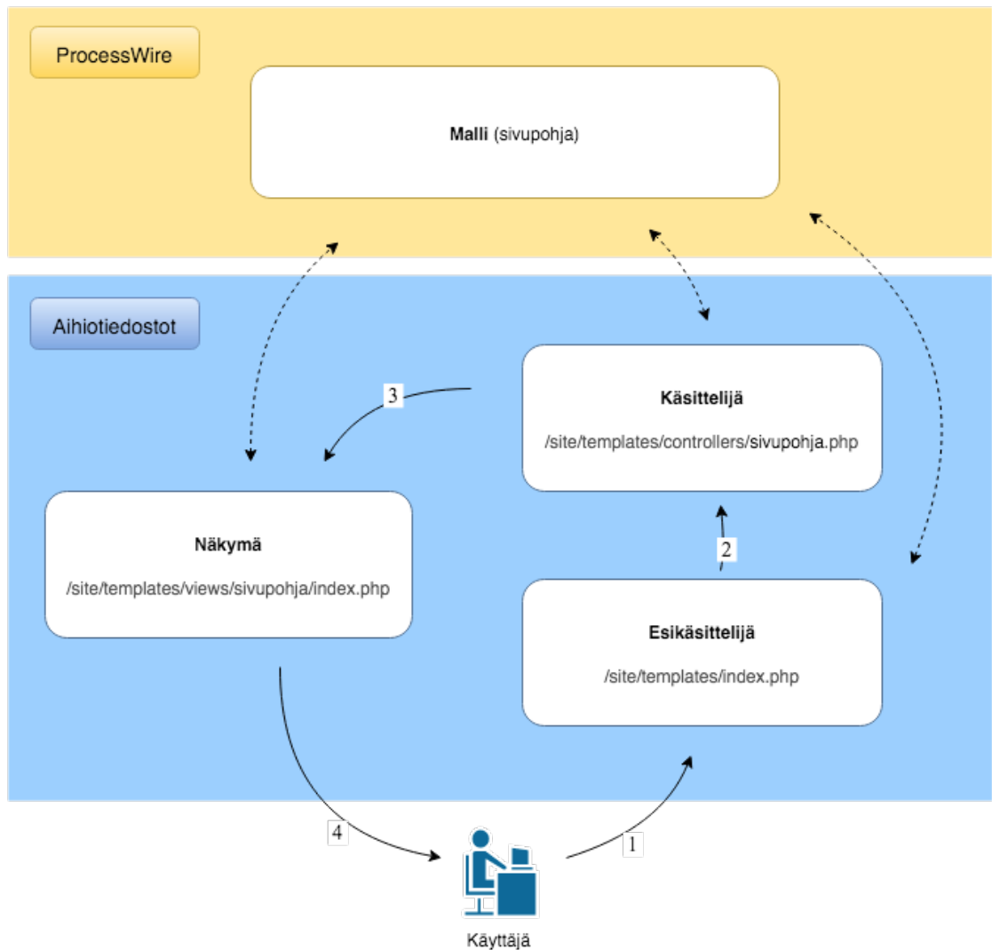
KAAVIO 18. Elementit ja niiden väliset interaktiot opinnäytetyön aihotasolla toteutettavassa MVC-mallin mukaelmassa. Katkoviivat kuvaavat mahdollista yhteyttä, nuolet viestien suuntaa. Nuoli molemmissa päissä viittaa kahdensuuntaiseen liikenteeseen.
