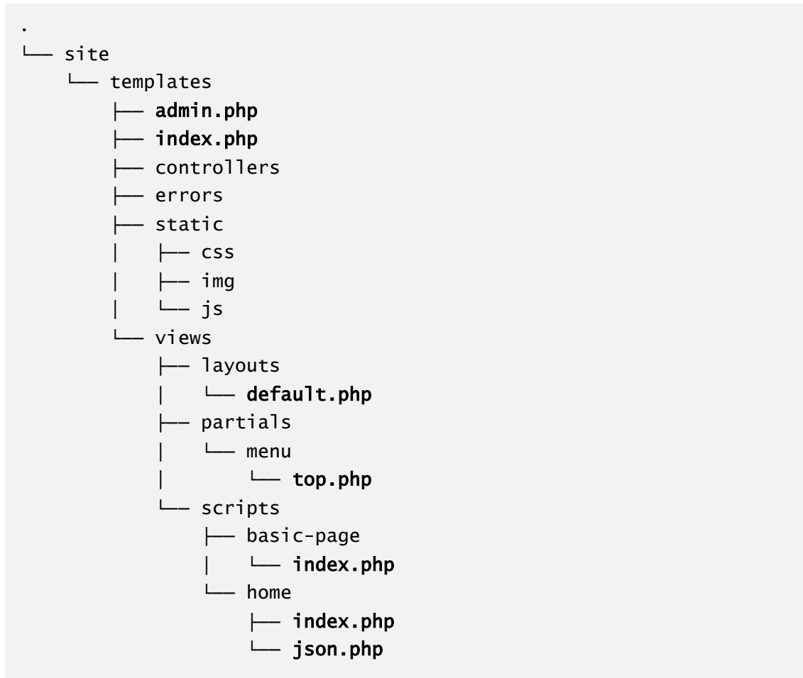
KAAVIO 19. MVC-esimerkkitoteutuksen hakemistorakenne.
