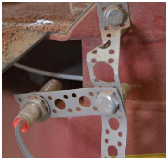
Kuva 4. RS 100 piensiemenvittimeen asennettu kierroslukumittari.
