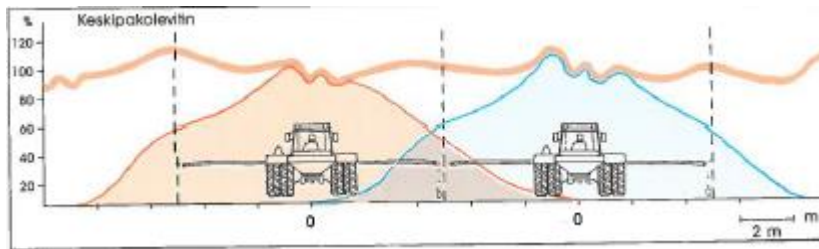
Kuvio 3. Keskivakolevittimen levityskuvio ja lomittain ajo (Heikkilä ym. 1991, 17).
