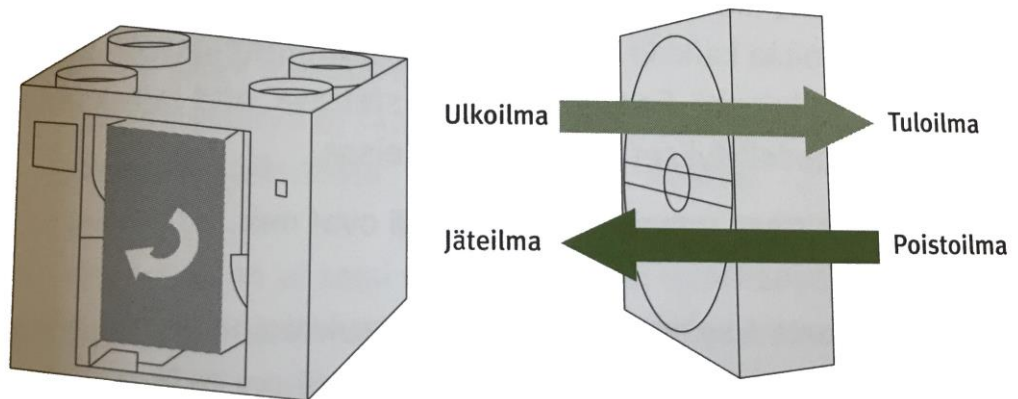
KUVIO 3. Pyörivän lämmönsiirtimen toimintaperiaate (Lappalainen. 2010, 64)
