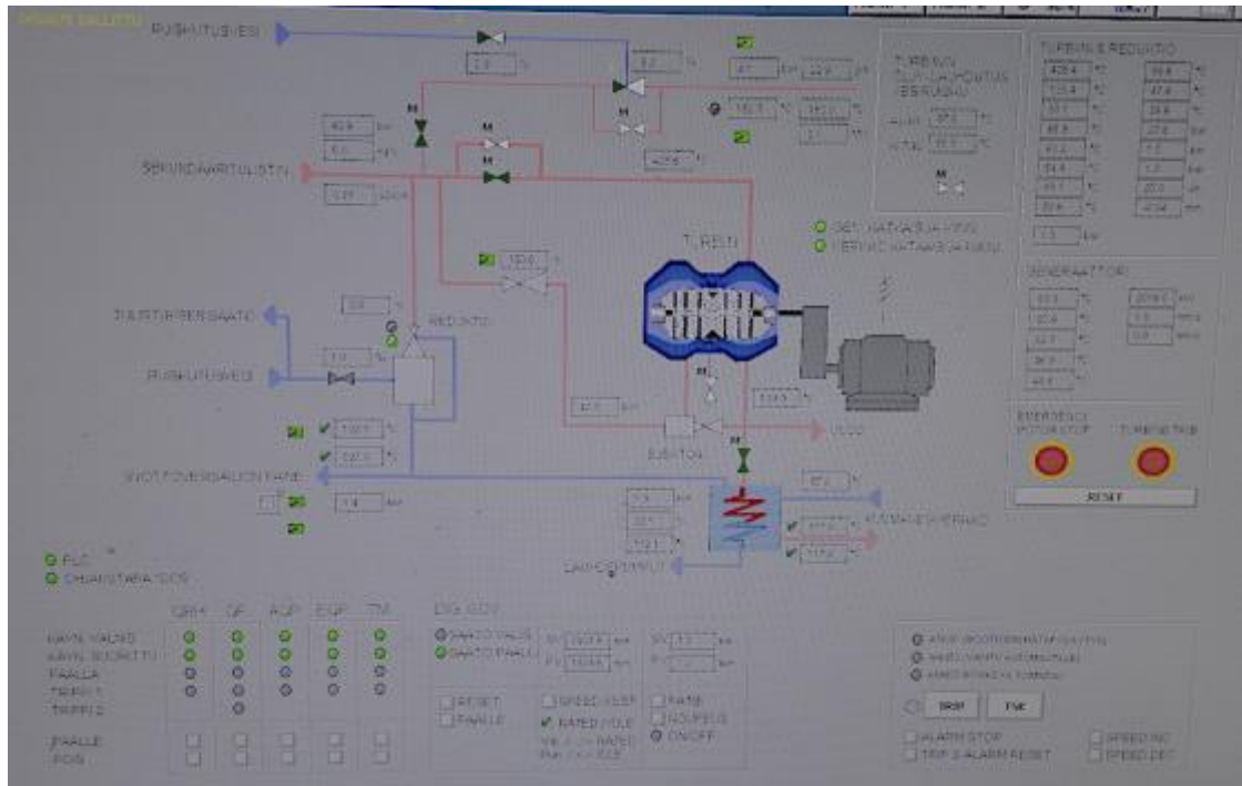
Kuvio 15. Turbiini (Voimalaitoksen DCS)
