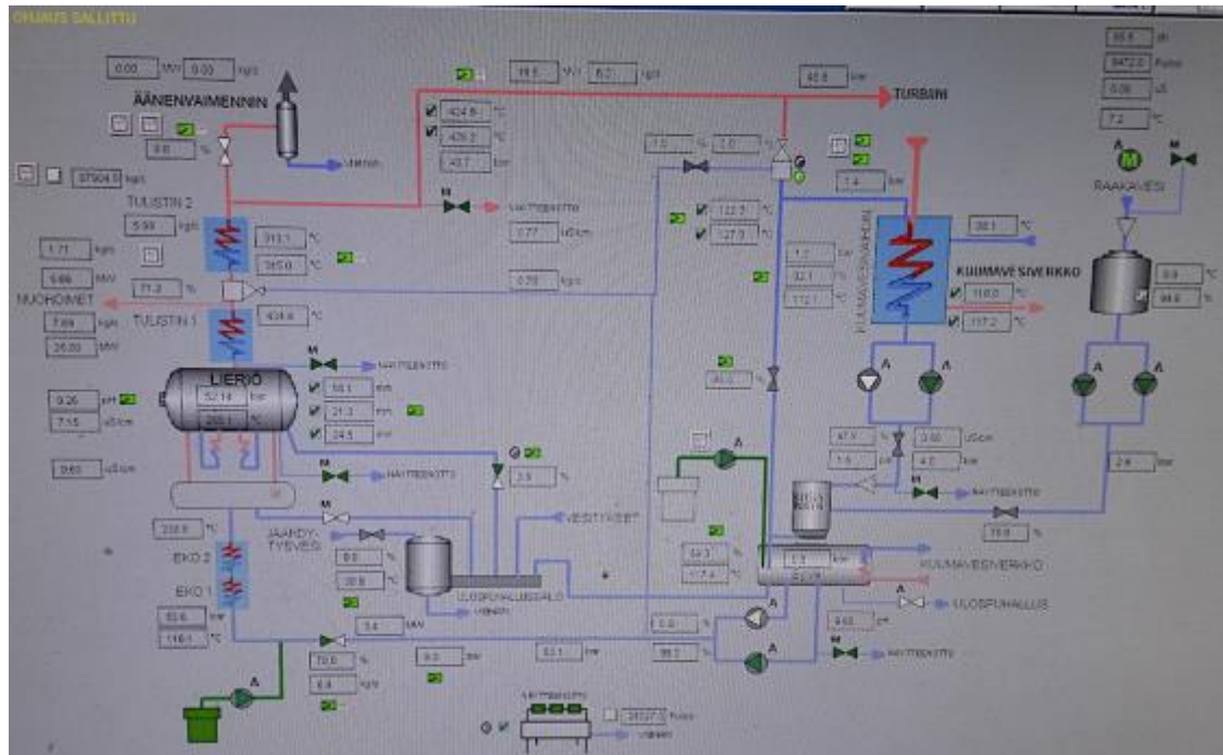
Kuvio 12. Vesi- ja höyryprosessi (Voimalaitoksen DCS)
