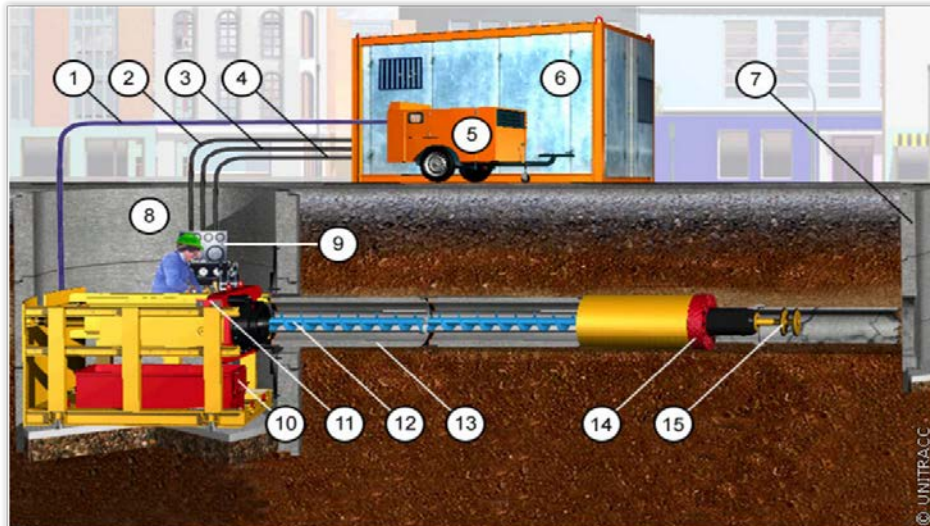
Kuvio 10. Mikrotunneloivan pakkosujutuksen havainnekuva. 1:Paineilmalinja, 2-4:Hydrauliletkuja, 5:Paineilmakompressori, 6:Hydrauliyksikkö, 7:Lopetuspiste, 8:Aloituspiste, 9:Ohjausyksikkö, 10:Lietteen keräysastia, 11:Työntölaite, 12:Ruuvikuljetin, 13:Asennettu mikroputki, 14:Tunnelointipää ja -pään murskain, 15:Pilottiputki ja tiivistyslaipat.
