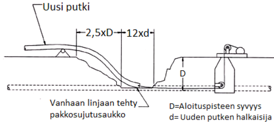
Kuvio 15. Esimerkki lähtökaivannon koon mitoittamiseksi pakkosujutettaessa jatkuva putkimateriaalia. (alkup. kuvio ks. Guideline for pipe bursting 2012, 21, muokattu.)
