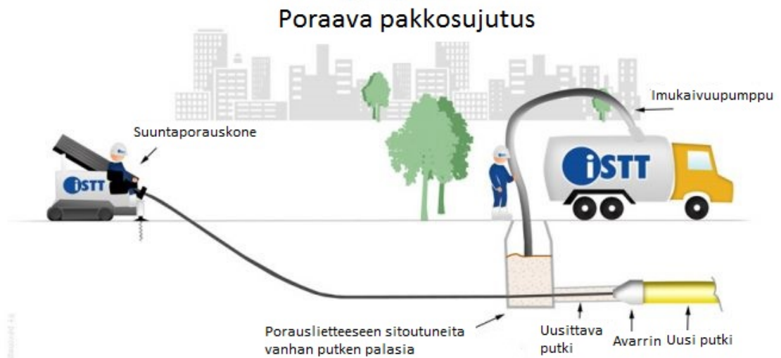
Kuvio 9. Poraavan pakkosujutuksen havainnekuva. (alkup. kuvio ks. Pipe Reaming n.d. ISTT, muokattu.)
