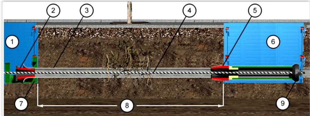
Kuvio 8. Tunkkaavan pakkosujutuksen havainnekuva. 1:Lopetuspiste, 2:Vanhan putken hajoituskartio, 3:Vanha putkimateriaali, 4:Vetovaijeri, 5:Sovitinpää, 6:Aloituspiste, 7:vetokoneen tuenta, 8:<100m, sisältäen mahdolliset välikaivannot, 9:Vetolevy (alkup. kuvio ks. Pipe extraction process for the replacement of cast iron pipelines (Hydros System) n.d.)
