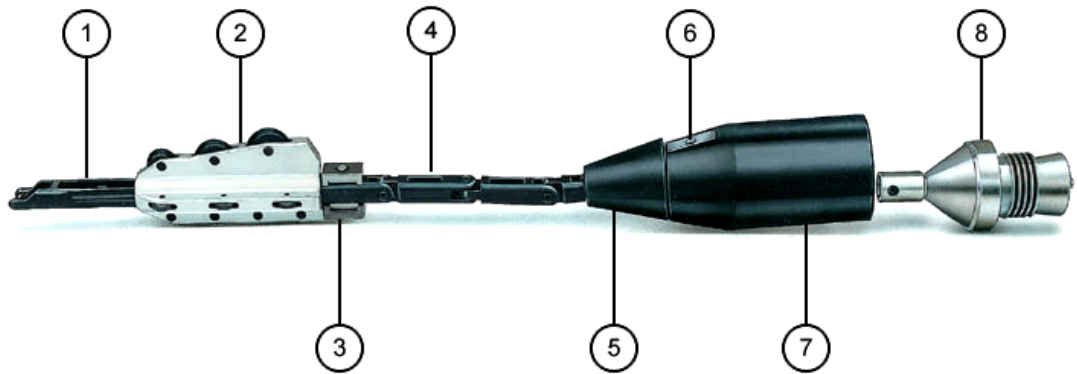
Kuvio 7. Halkaisevassa menetelmässä käytettäviä pakkosujutuspuun laitteita. 1:Veto- tangon pää, 2:Leikkaustyökalu, 3:rikotutyökalun tuki tankoon, 4:välitangot, 5-7:Avarrin, 8:Vetopää. (alkup. kuvio ks. Rehabilitation and Maintenance of Drains and Sewers n.d.)
