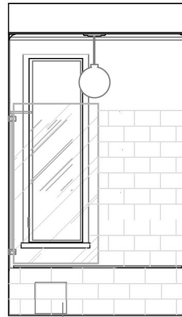
IKKUNASEINÄ TARKISTUSLUUKKU
