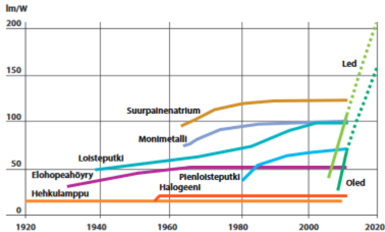
Kuvio 6. Valaisimien valontuottojen kehitys (RT 75-11118 2013, 2)
