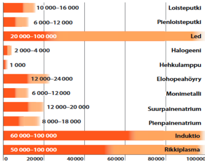
Kuvio 3. Valaisimien käyttötunnit (RT 75-11118 2013, 4.)
