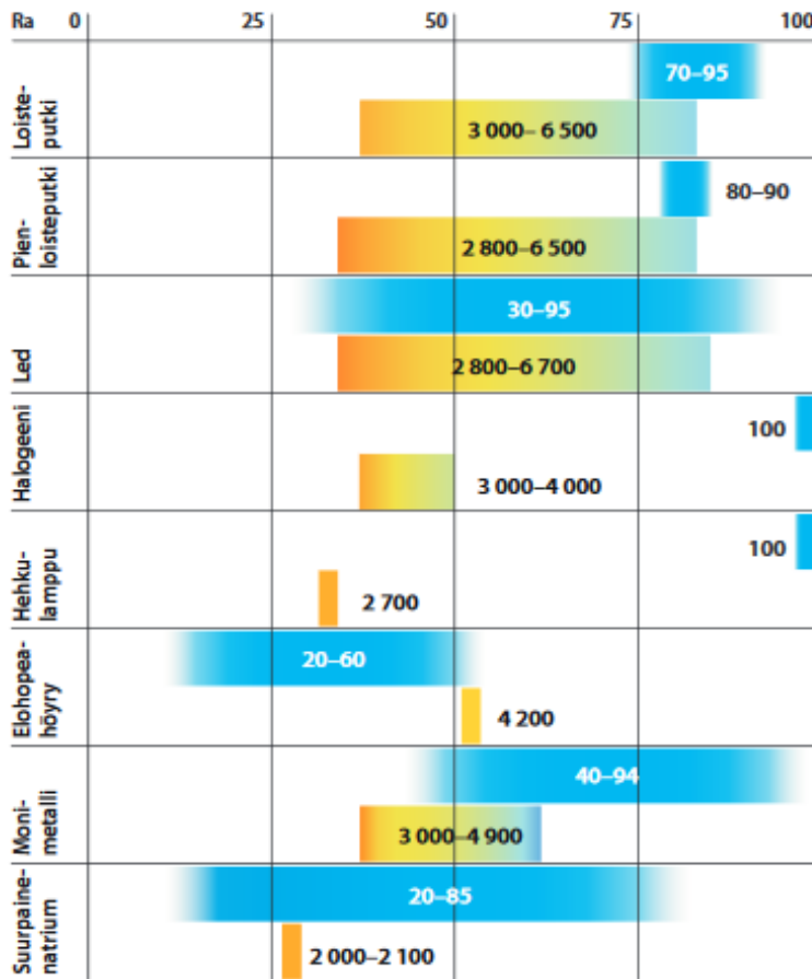
Kuvio 4. Erilaisten valaisimien Ra-arvoja sekä väriämpötiloja (RT 75-11118 2013, 4)
