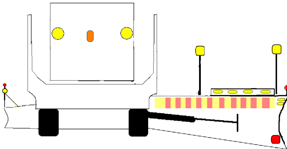
Kuva 47. Opinnäytetyön viitteellinen suositus sivuaurallisen aurausyksikön havaittavuuden parantamiseksi.
