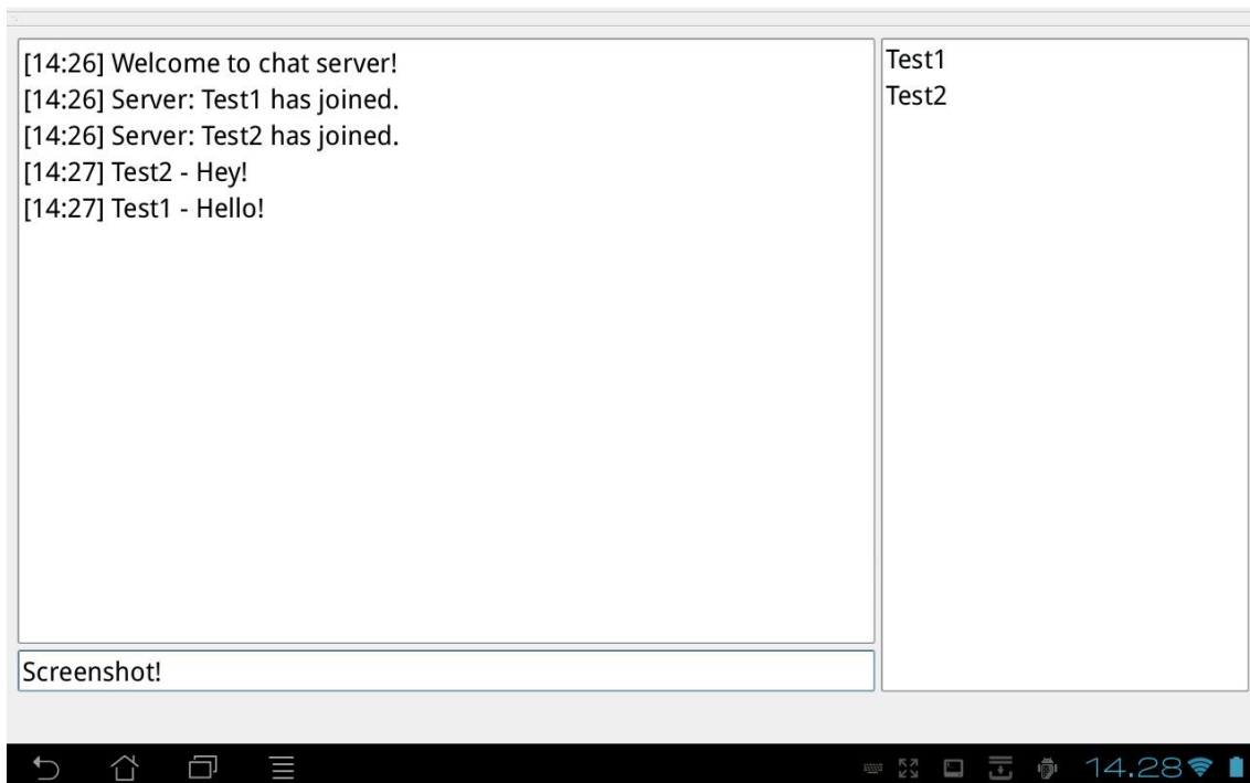
KUVA 7. Yksinkertainen keskusteluohjelma
