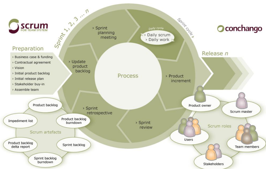
KUVA 2. Scrum-prosessi (Bird 2006)
