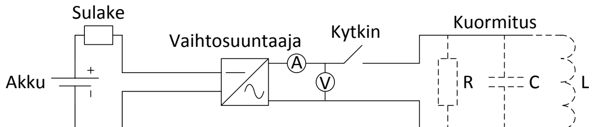
KUVIO 2. Mittauksissa käytetty koejärjestely.
