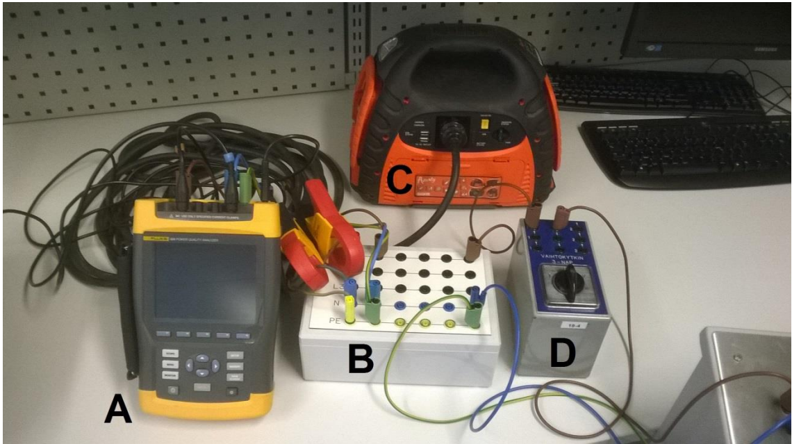
KUVA 4. Mittauksissa käytetty kytkentä (A on Fluke 435 mittalaite, B on jakolevy, C on tutkimuskohteena ollut invertterti ja D on kytkin).
