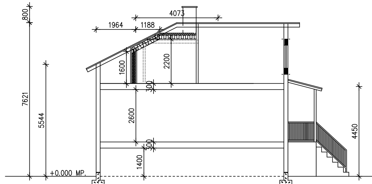
LEIKKAUS B-B 1:100
