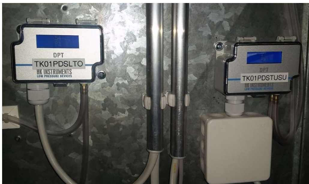
Kuva 7. Tuloilmakoneeseen 1 2010-luvulla lisättyjä mittauslaitteita. Vasemmalla paine-eromittari lämmöntalteenoton yli ja oikealla paine-eromittari tuloilmasuodattimen yli.
