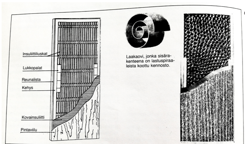
KUVA 6 Kuitulevyrakenteisen Inso-oven valmistus alkoi 1945. Koivunlastukierukkarakenteinen Inso-Rol-ovien valmistus alkoi 1950
